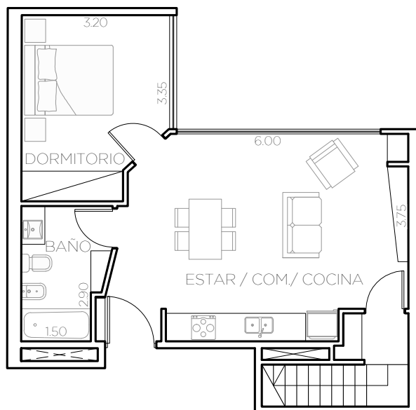
PLANTA 1
