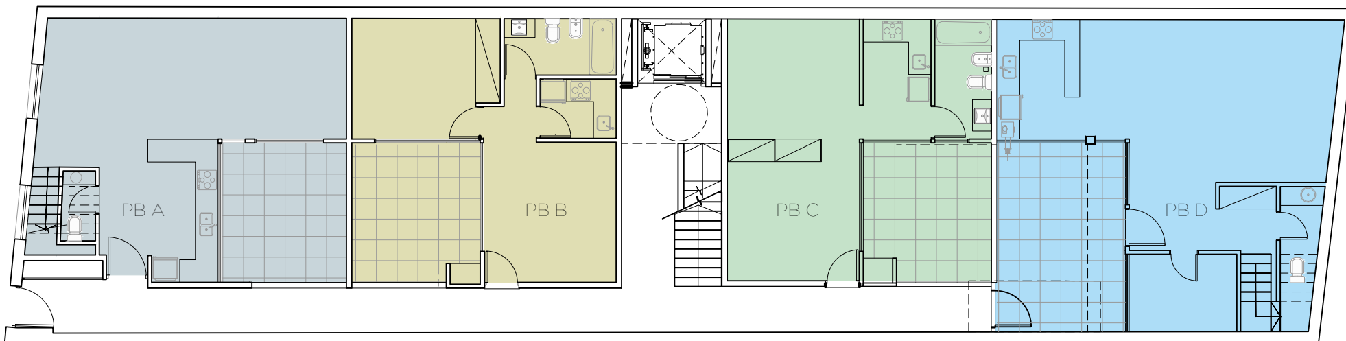
PLANTA BAJA
