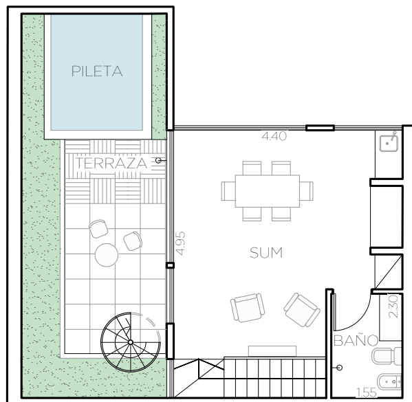
PLANTA TERRAZA
