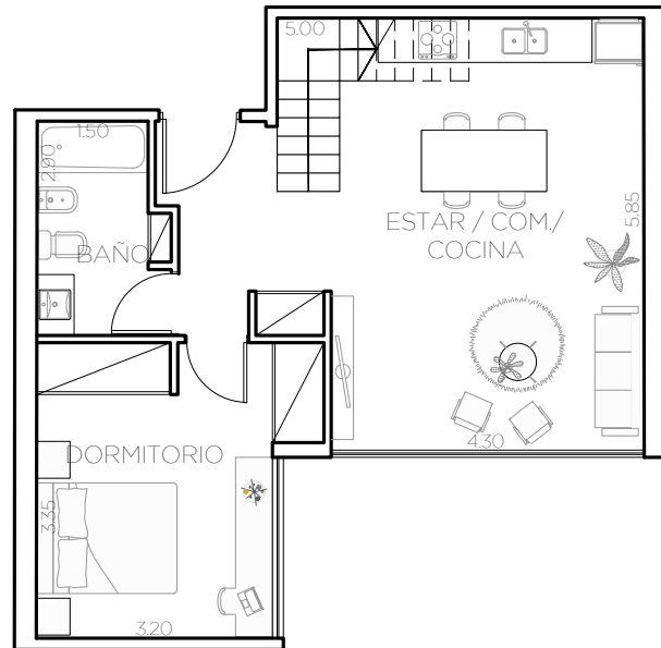
PLANTA 1
