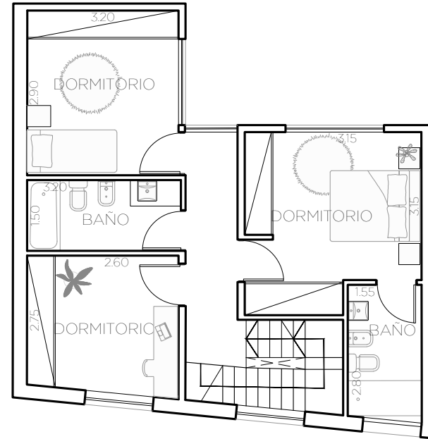
PLANTA 2
