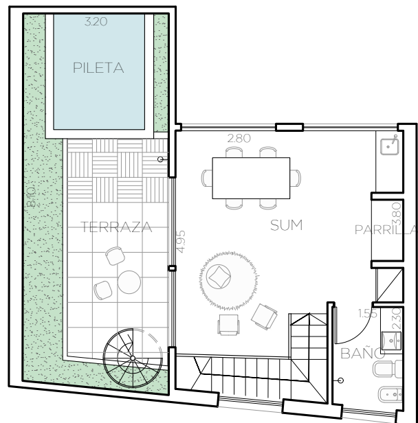
PLANTA TERRAZA
